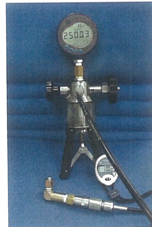
耐水壓試驗
