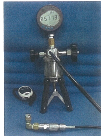
耐水壓試驗
